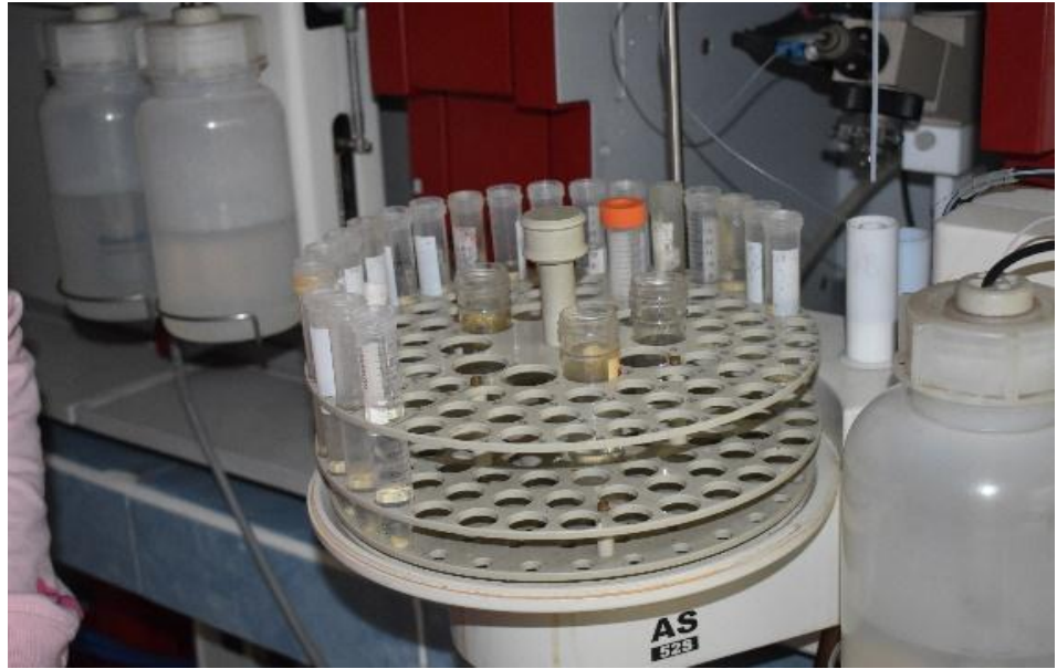
Gambar 9. Memasukkan sampel ke alat Atomic Absorption Spectrophotometer (AAS)
