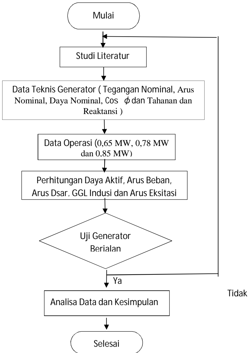
Gambar 3.2 Diagram Alir Pengambilan dan Pengolahan Data
