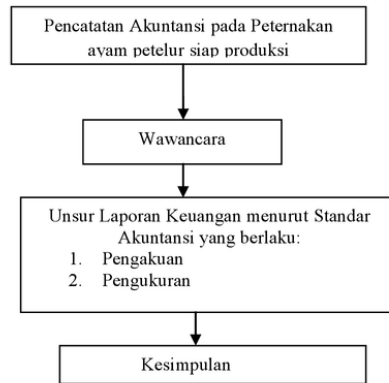
Gambar 1 Kerangka Konseptual
