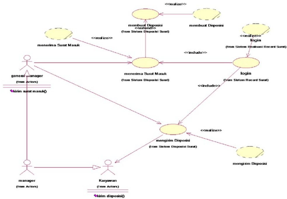
Gambar 3. Sistem Realisasi Disposisi
