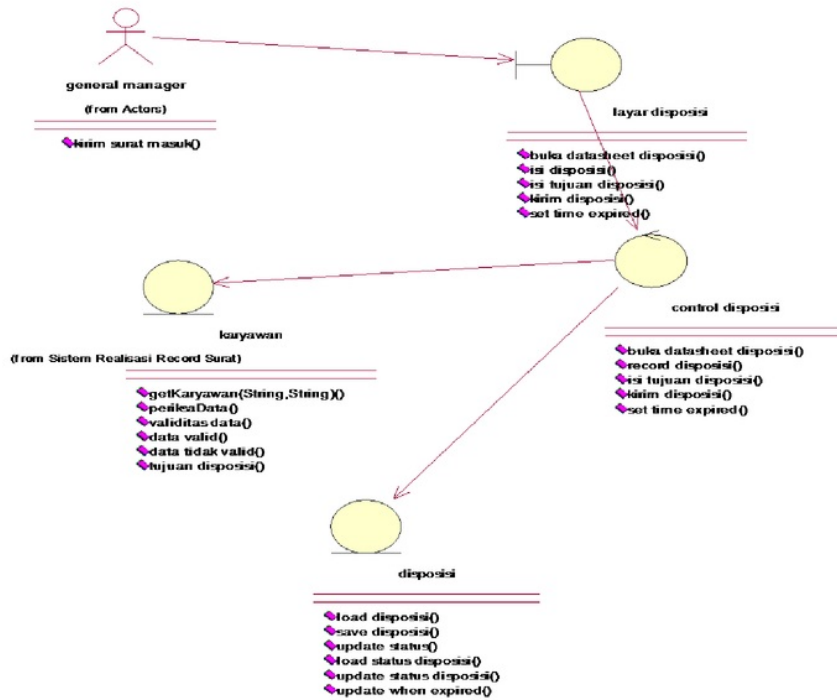
Gambar 5. Hubungan Class Disposisi
