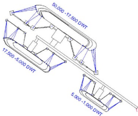
Gambar3: Layout studi
