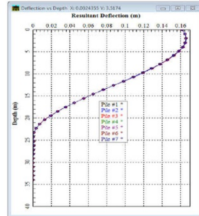
Deformasi Lateral: 16.2 cm Alternatif 2 (Dia. 800, 16 mm)
