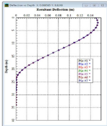
Deformasi Lateral: 15.0 cm Alternatif 1 (Dia. 900, 12 mm)
