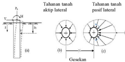
Gambar 1: distribusi tekan pada lateral tiang pancang
