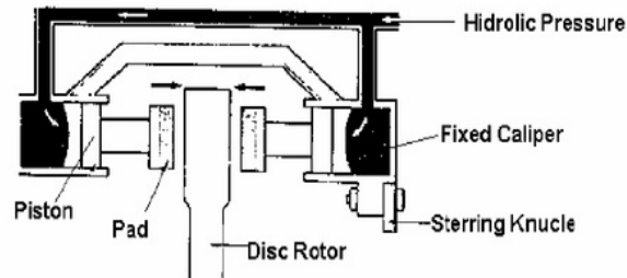
Gambar 2. 7Kaliper jenis Fixed Caliper ( sumber:sumber: Dadang,Jurnal Konversi Energi dan Manufaktur UNJ))
