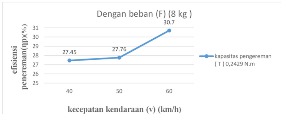
Gambar 4. 1grafik kapasitas pengereman dan variasi kecepatan pada beban 8 kg
