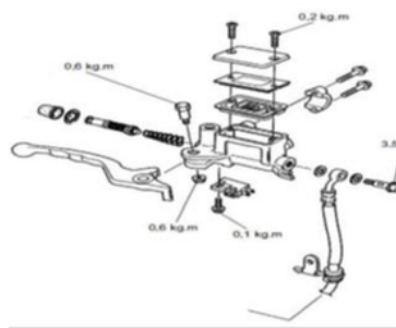
Gambar 2. 3 Master Silinder, (sumber: Dadang, Jurnal Konversi Energi dan Manufaktur UNJ)
