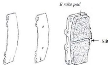
Gambar 2. 5 Pad Rem Cakram (sumber: Dadang, Jurnal Konversi Energi dan Manufaktur UNJ)
