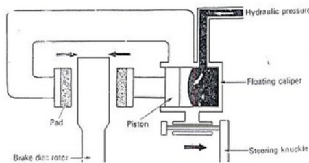
Gambar 2. 8Kaliper Jenis floating caliper (sumber: Dadang,Jurnal Konversi Energi dan Manufaktur UNJ)
