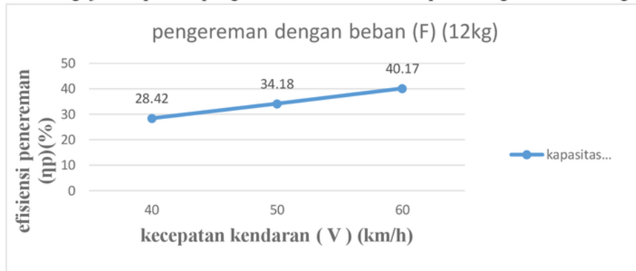
Gambar 4. 3 Grafik kapasitas pengereman dan variasi kecepatan pada beban 12 kg
