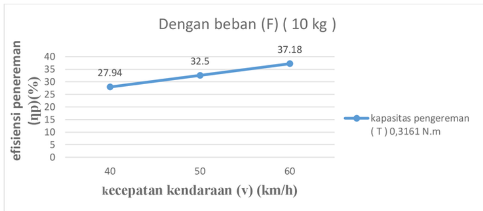
Gambar 4. 2grafik kapasitas pengereman dan variasi kecepatan pada beban 10 kg
