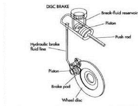
Gambar 2. 2 Rem, (sumber: Dadang, Jurnal Konversi Energi dan Manufaktur UNJ)
