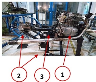
Gambar 3. 1 Alat uji rem cakram 1 (sumber: Laboratorium Universitas Muhammadiyah Surabaya)
