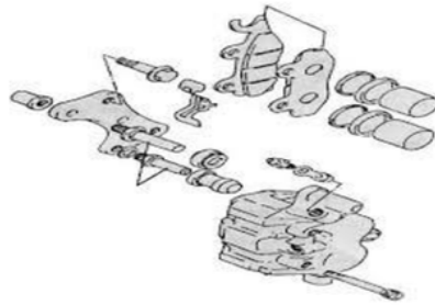
Gambar 2. 4Komponen kaliper (sumber: suratman, 2002:250)
