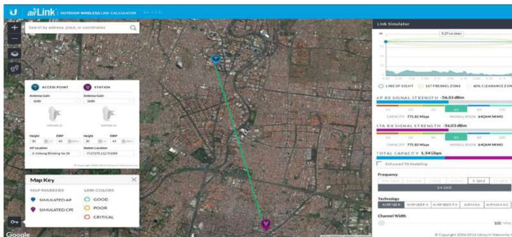
Gambar 8. Link Budget perangkat backhaul tier 3 (24Ghz)
