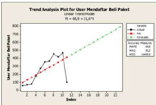
Gambar 3. Peramalan Linier
