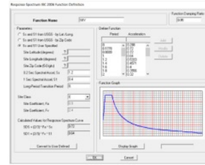
Gambar 12. Grafik respon spektrum Sumber : Dokumen P.T. Alien Bangun Nusantara
