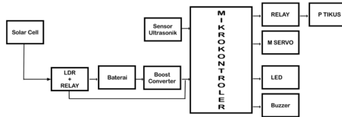
Gambar 3.1 Blok Diagram Sistem
