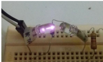
Gambar 4.6 Pengujian Sensor LDR
