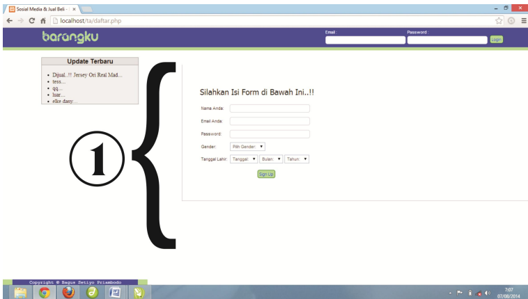
Gambar 4.2 : Halaman Daftar.php
