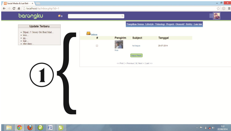
Gambar 4.4 : Halaman Inbox.php
