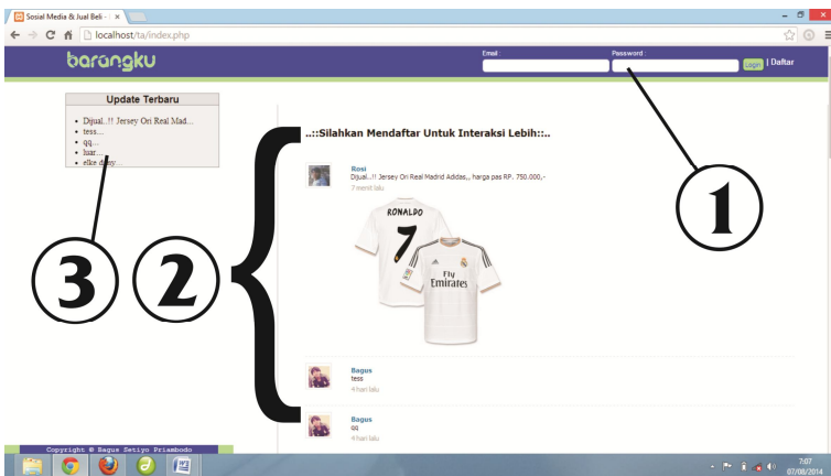
Gambar 4.1 : Halaman index.php
