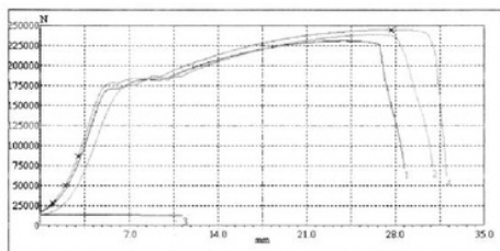
Gambar 3 Hasil Uji Tarik
