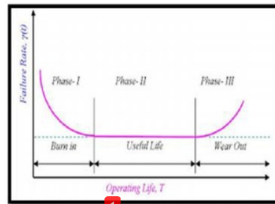
Gambar 1.2. Grafik laju kerusakan ( failure rate ) terhadap waktu
