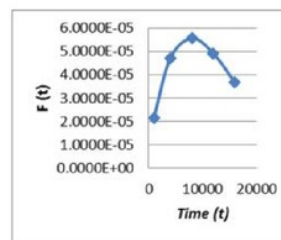
Gambar 4.1 Grafik f(t) terhadap t Inlet Valve
