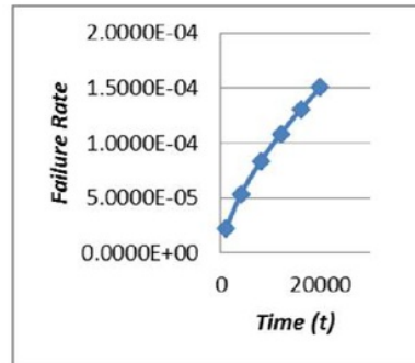
Gambar 3.3 Grafik \lambda(t) terhadap t Inlet Valve
