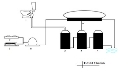
Gambar 3 Sistem Instalasi Biogas
