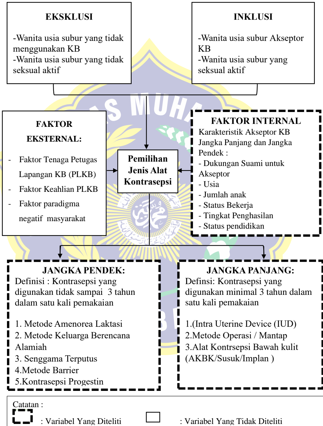
Gambar 3.1 Kerangka Konseptual
