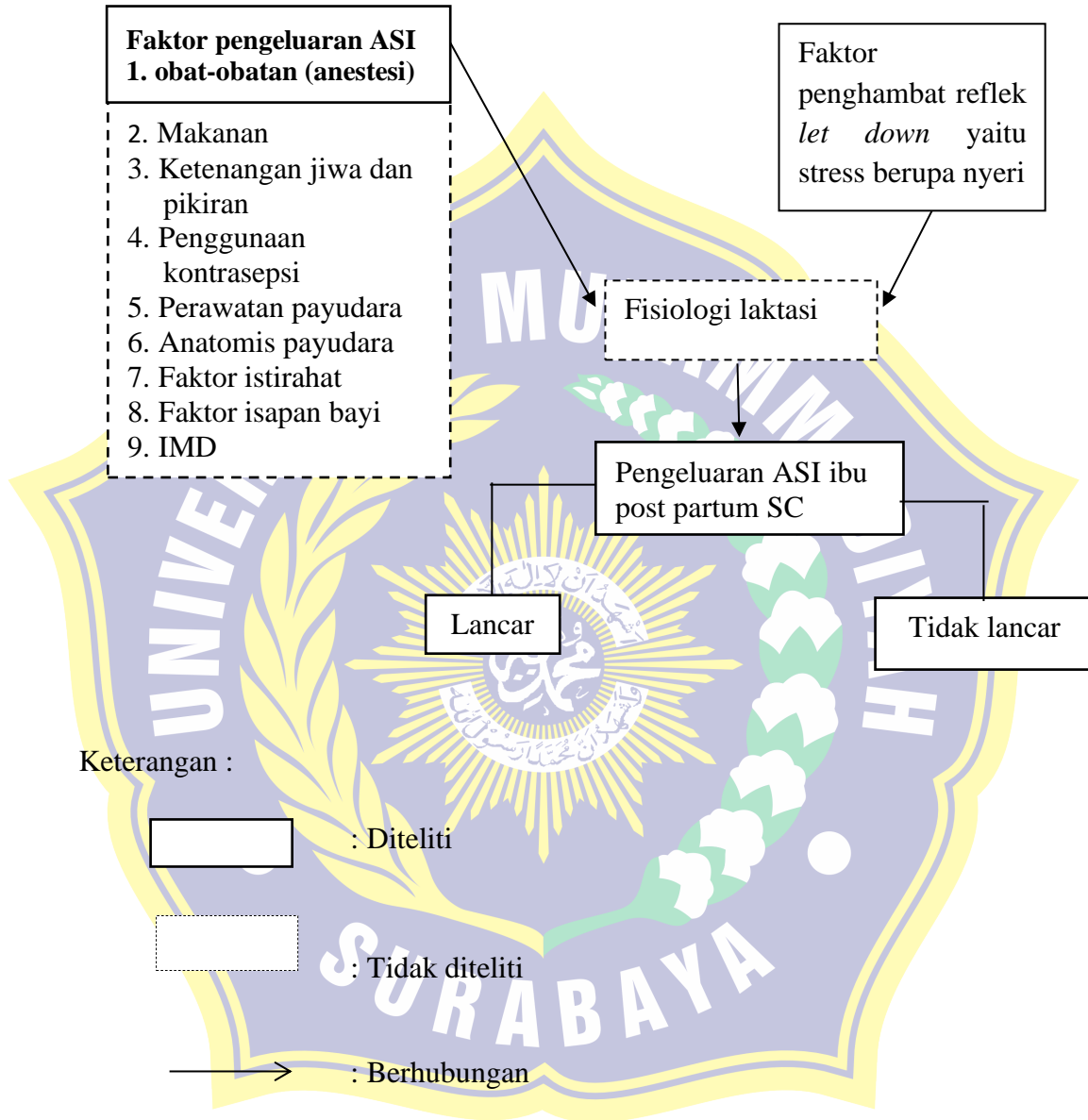
Gambar 3.1 Kerangka Konsep
