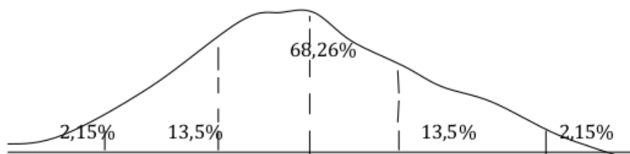
Bentuk dan daerah kurva normal
