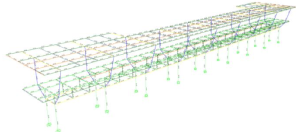
Gambar 11. Beban akibat suhu di ambil sebesar 20 °C Sumber : DokumenP.T. Alien Bangun Nusantara
