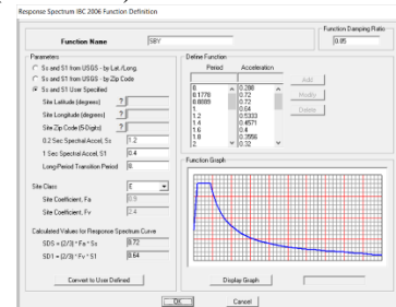
Gambar 12. Grafik responspektrum Sumber : DokumenP.T. Alien Bangun Nusantara
