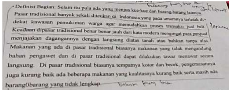
Gambar 3: Definisi Bagian
