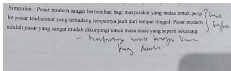
Gambar 1: Simpulan Singkat
