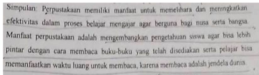
Gambar 2: Simpulan Lengkap
