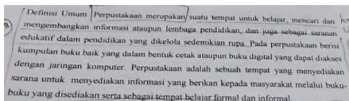
Gambar 4: Definisi Umum
