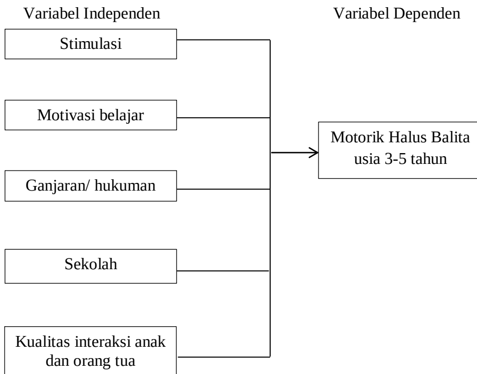
Gambar 3.1 Kerangka Konsep Faktor-faktor yang Mempengaruhi Motorik Halus Balita usia 3-5 Tahun
