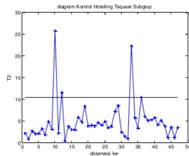
Gambar 3. Plot Kontrol T^2 Hotelling Data Juli 2007
