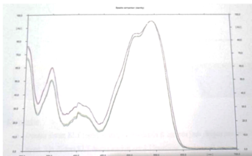
Gambar 2. Identifikasi dan purity Rhodamin B
