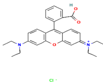
Gambar 1. Struktur Rhodamin B
