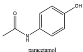
Gambar 1. Rumus kimia parasetamol
