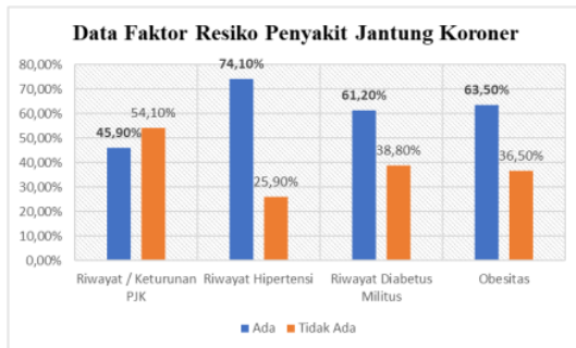
Gambar 1. Diagram Data Faktor Penyakit Jantung Koroner
