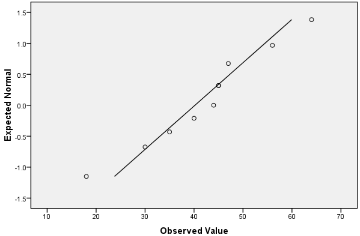
Normal Q-Q Plot of MENGABAIKAN
