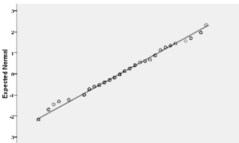
Normal Q-Q Plot of V.Penyediaan diri
