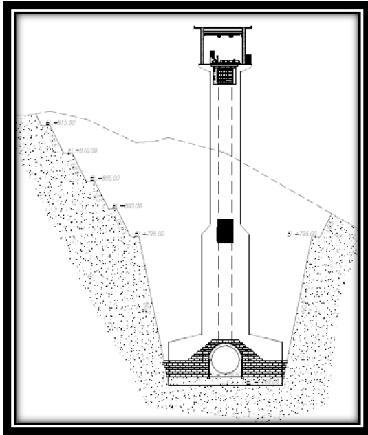
Gambar 2.2.2: penampang melintang portal terowong Sumber : Data Teknik PT Brantas Abiprava (Persero) 2018
