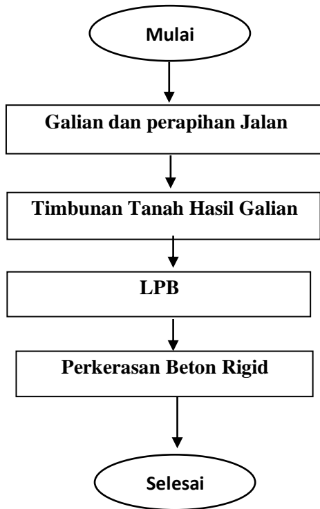
Gambar 2.2.1: Bagan Alir Pekerjaan Persiapan
