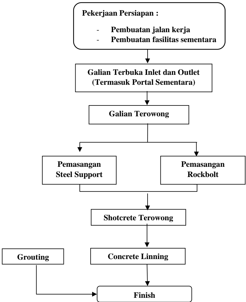
Gambar 2.1: Bagan Alir Pekerjaan Terowongan Sumber : Data Teknik PT Brantas Abipraya (Persero) 2018
