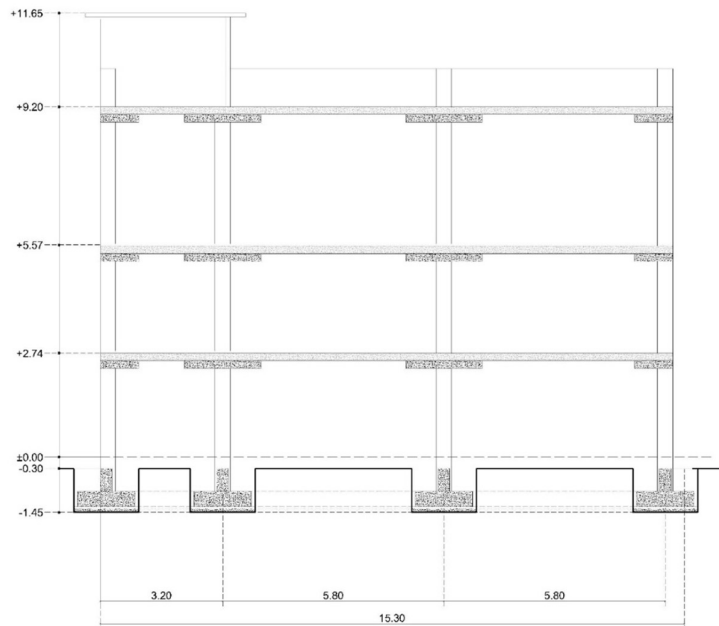
PORTAL A-A 1 SKALA 1 : 100
