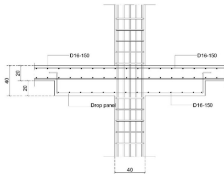
POT.1 SKALA 1:25
