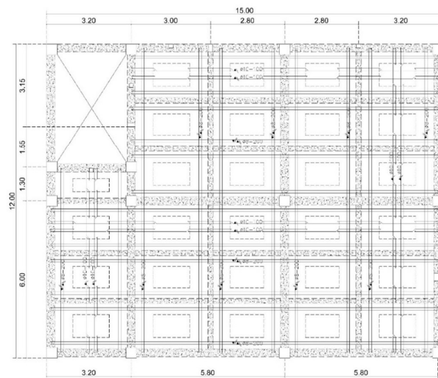
RENCANA PENUL. LANTAI LT. 3 SKALA 1 : 100
