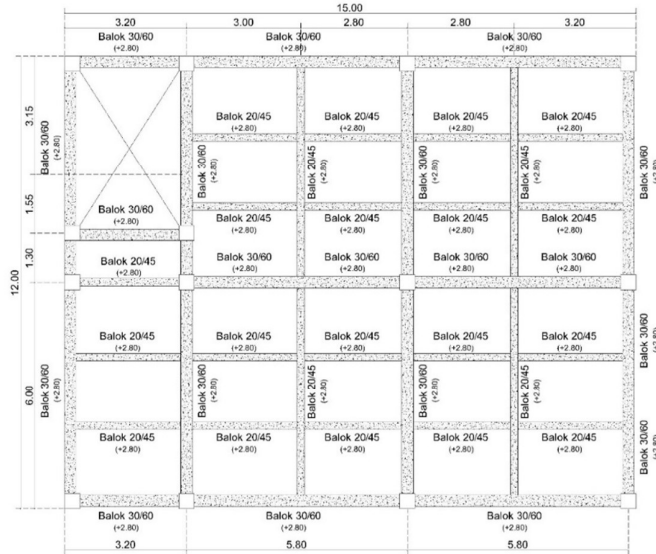
DENAH BALOK LT. 2 - 4 SKALA 1 : 100
