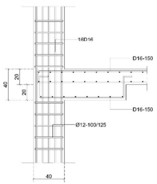
POT.2 SKALA 1 : 25
