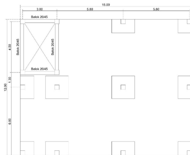
DENAH BALOK LANTAI 1 - 4 SKALA 1 : 100
