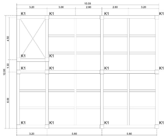
DENAH KOLOM LT. 2 - 4 SKALA 1 : 100
