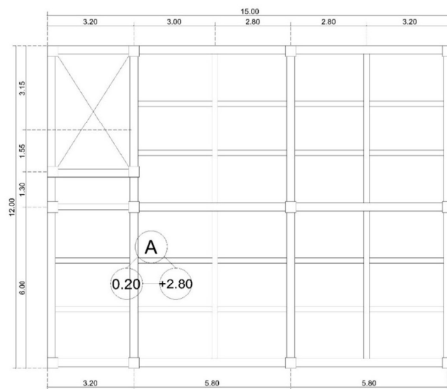
DENAH PLAT LT. 2 SKALA 1 : 100
