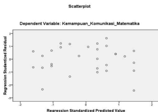
Gambar 1. Hasil Heteroskedastisitas
