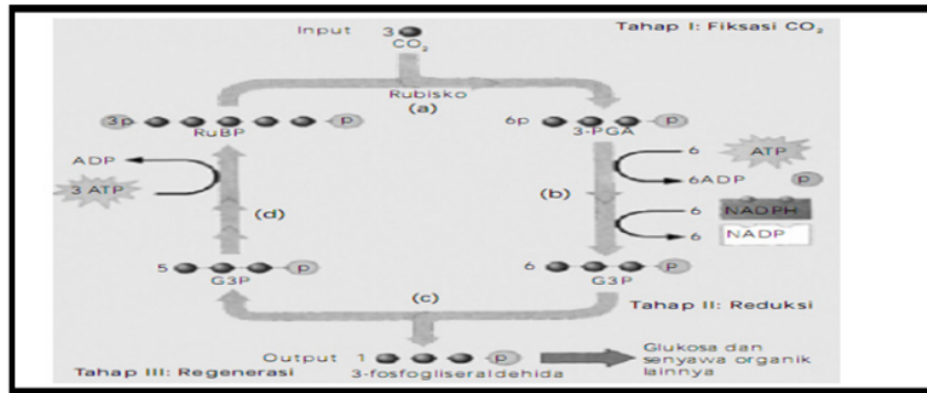
siklus Calvin-Benson
