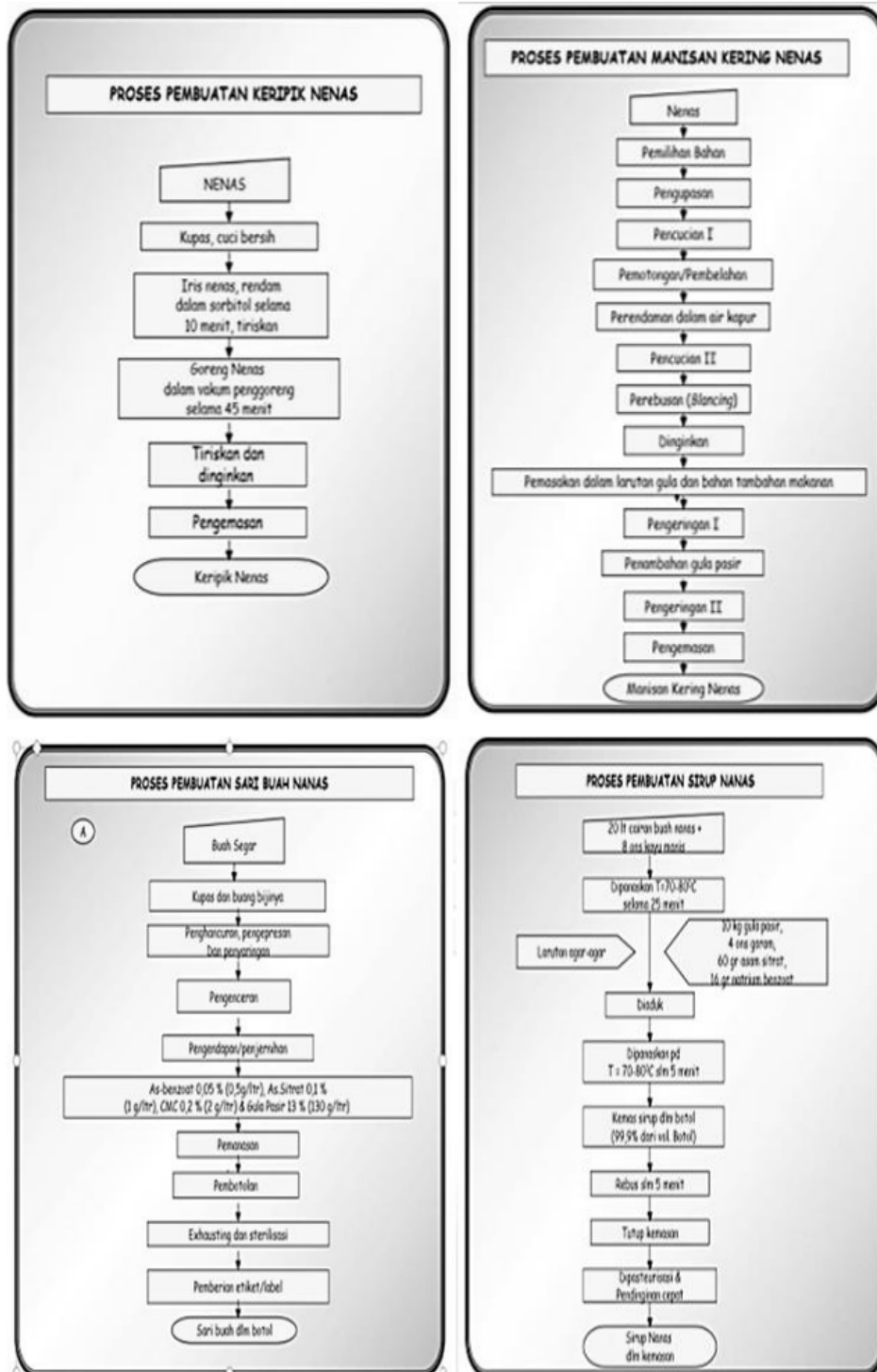
Gambar 7. Alur Proses Produksi Produk
