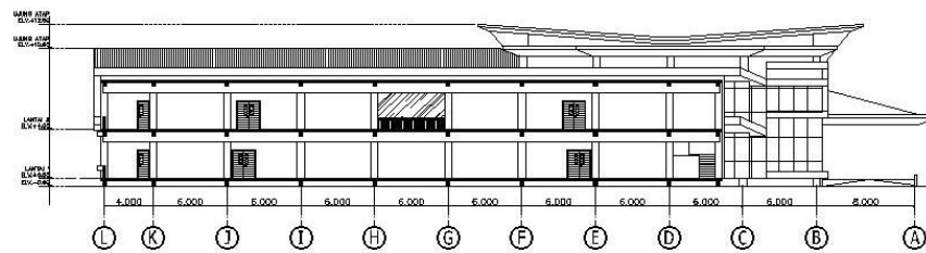
POTONGAN B-B
