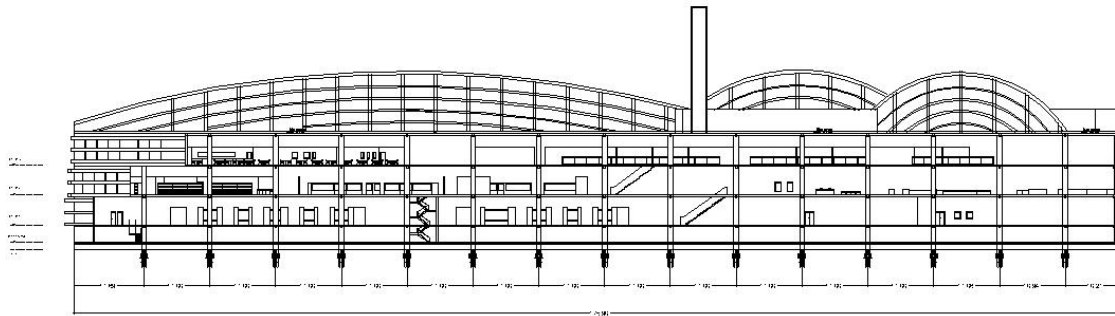
POTONGAN A-A MUSEUM BIOTA LAUT KENJERAN SKALA: 1:500
