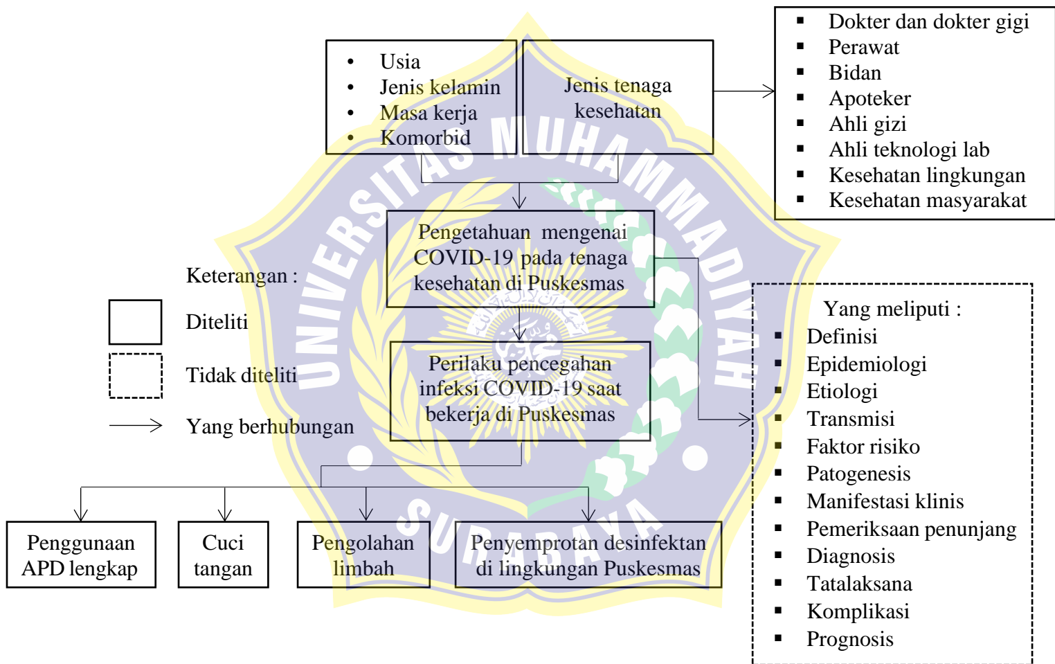
Gambar 3.1 Kerangka Konseptual
