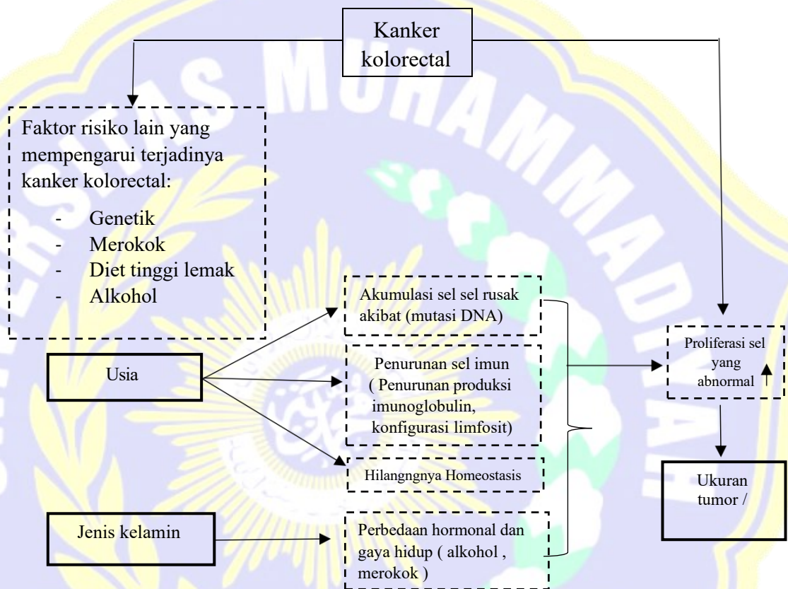
Gambar 3.1 : Kerangka Konseptual
