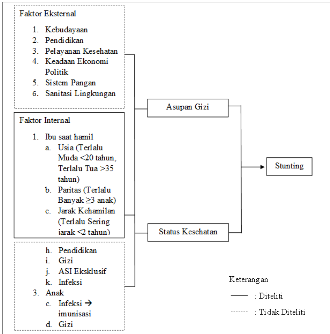
Gambar 3.1 Kerangka Konsep
