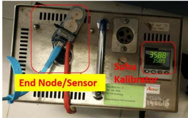
Gambar 5. Proses Perbandingan Sensor Suhu dengan suhu standar
