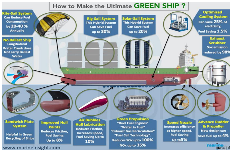
Gambar 2. Teknologi solusi dalam green ship technology Sumber gambar: marineinsight
