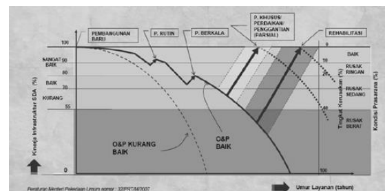
Gambar 2. Korelasi antara Kinerja Infrastruktur, Pemeliharaan dan umur layanan. (Sumber Dirjen SDA, Operasi dan pemeliharaan Sumber Daya Air, 2011)
