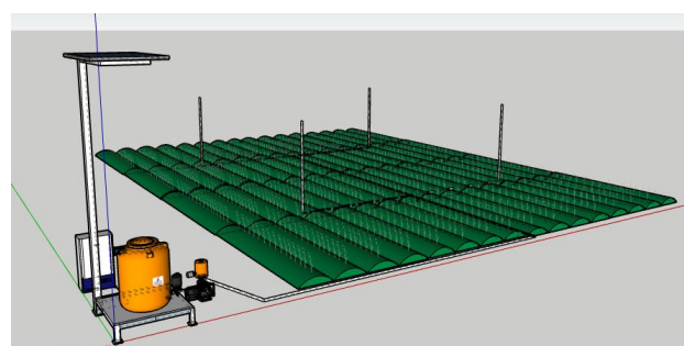
Gambar 6. Tampak Samping Alat Penyemprot Hama
