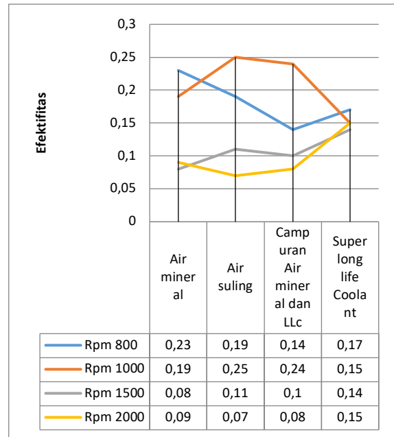
Gambar 5. Perbandingan hasil efektivitas penyerapan panas radiator
