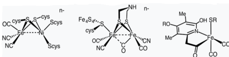
Gambar 2.2 Struktur situs aktif dari tiga jenis enzim hydrogenase.
