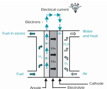
Gambar 6.2. Fuel cell jenis PEM
