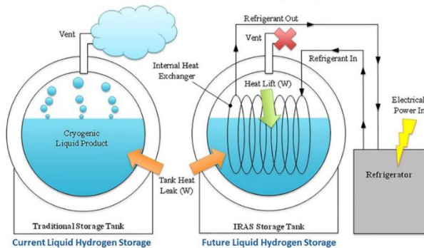
Gambar 4.4 Teknologi tabung gas hidrogen menghilangkan loss boil-off hidrogen
