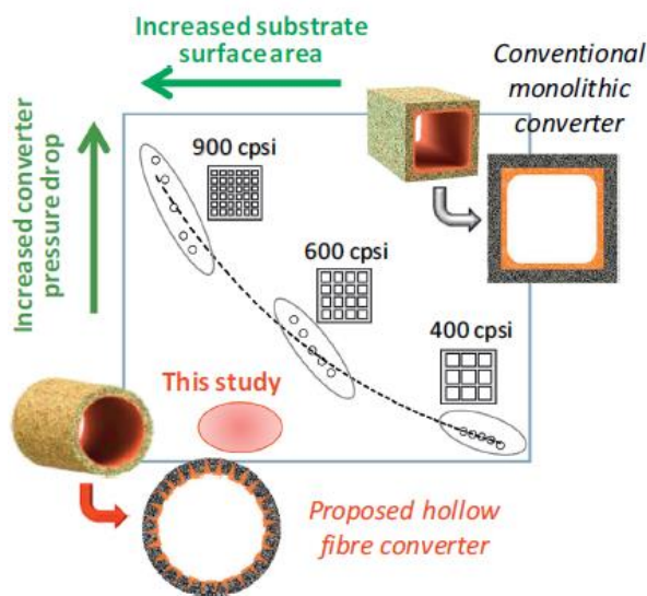
Gambar 2. Perbandingan skematik diagram antara conventional catalytic convertor dengan hollow fibre converter . Diadaptasi dari (Mahyon et al., 2019)
