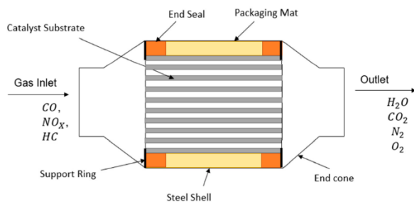
Gambar 1. Automobile catalytic converter . Diadaptasi dari (Kritsanaviparkporn et al., 2021)
