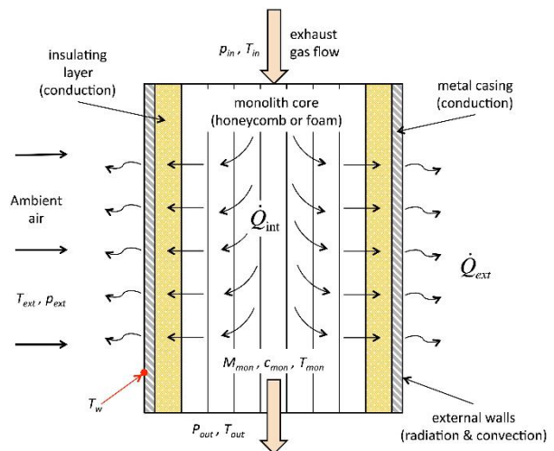
Gambar 3. Skematik diagram untuk aliran dan proses perpindahan panas pada catalyst core . Diadaptasi dari (Gambarotta et al., 2019)
