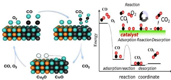
Fig. 5. Adsorption-desorption gas CO melalui katalis copper oxide . Diadaptasi dari (Dey & Chandra Dhal, 2020)
