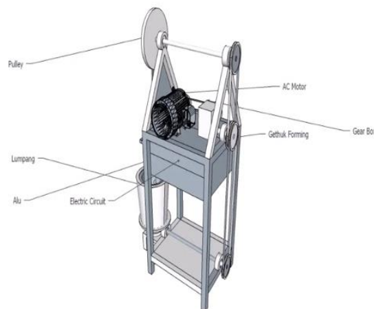
Gambar 2 Bagian-bagian pada alat penumbuk udang rebon
