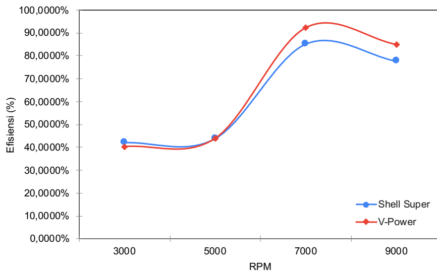
Gambar 5. Grafik Hubungan Putaran Mesin dengan Efisiensi Thermal
