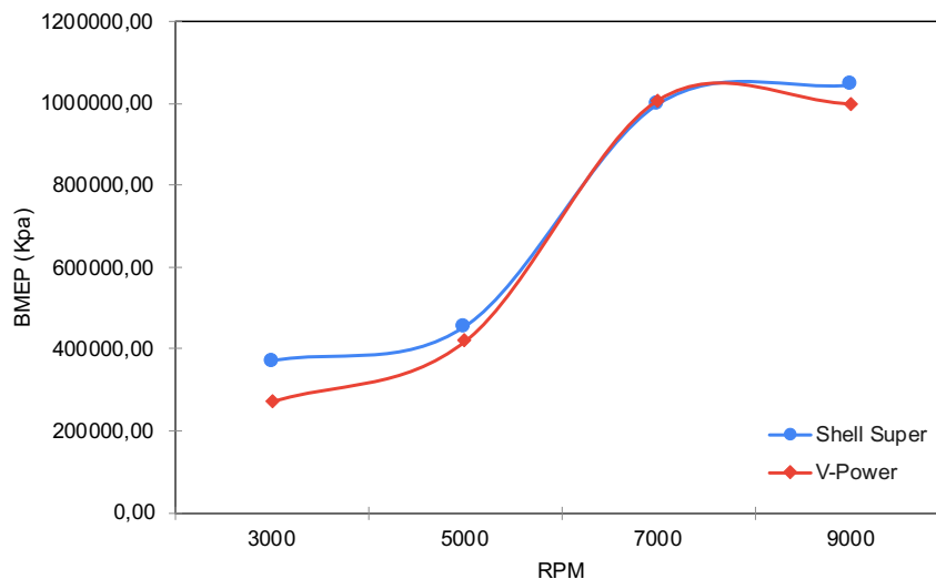
Gambar 4. Grafik Hubungan Putaran Mesin dengan BMEP
