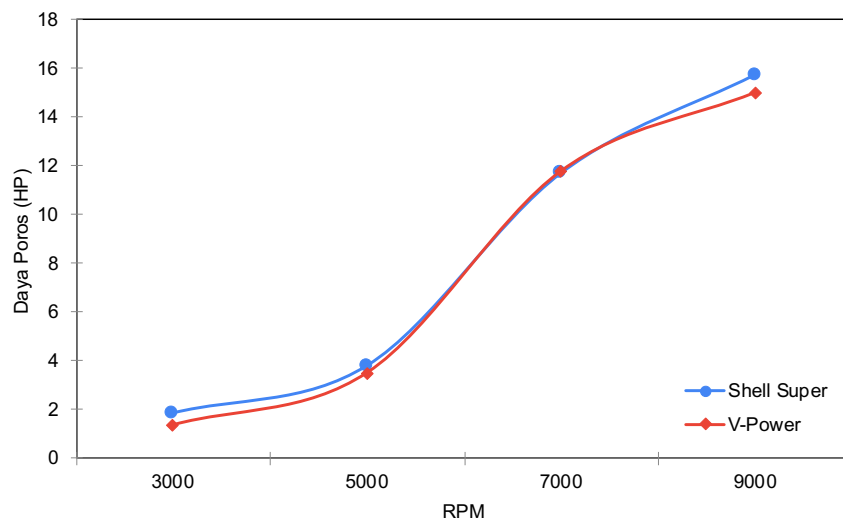
Gambar 2. Grafik Hubungan Putaran Mesin Dengan Daya Poros
