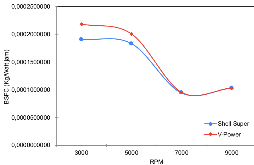
Gambar 3. Grafik Hubungan Putaran Mesin dengan BSFC
