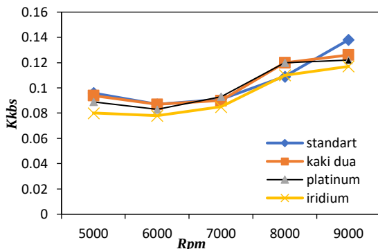
Gambar 4. Grafik hubungan KKBS dengan tipe beberapa busi terhadap RPM
