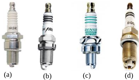
Gambar 1. Beberapa jenis busi (a). standar (NGK C7HSA), (b). platinum (NGK CR7HGP), (c). iridium (DENSO IUF24) dan (d). kaki dua (Fukukawa FKW-C7E)
