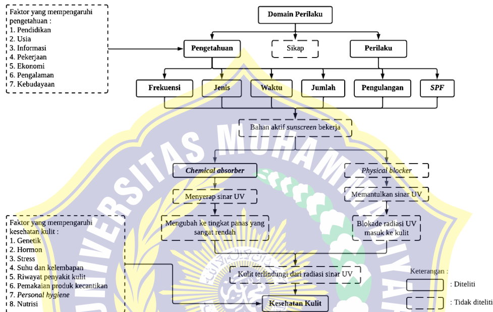
Gambar 3. 1 Kerangka Konseptual
