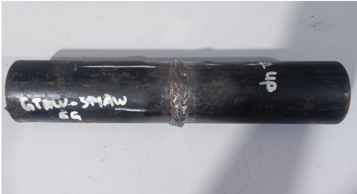
Obyek Uji (Pipa OD = 59,7 mm, Tebal = 8 mm)
