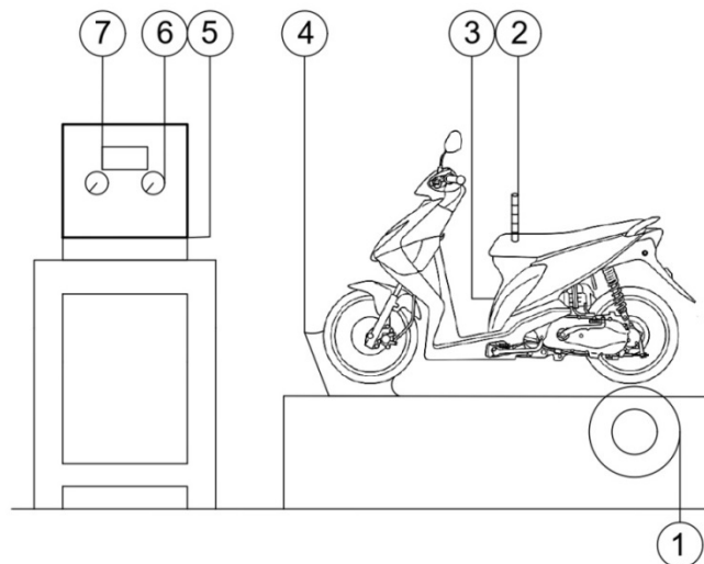
Gambar 1. Skema Pengujian Menggunakan Dynotest
