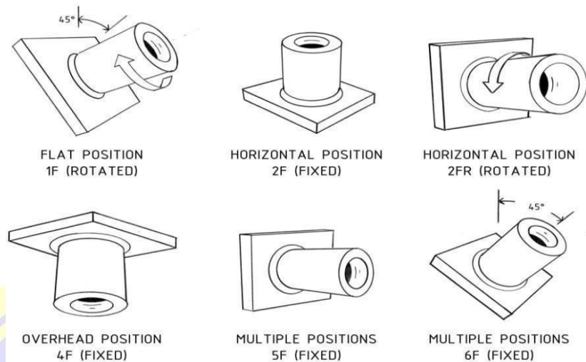
Gambar 2. Sambungan Fillet Pipa
