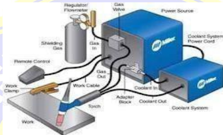
Gambar 1. Peralatan Las GTAW
