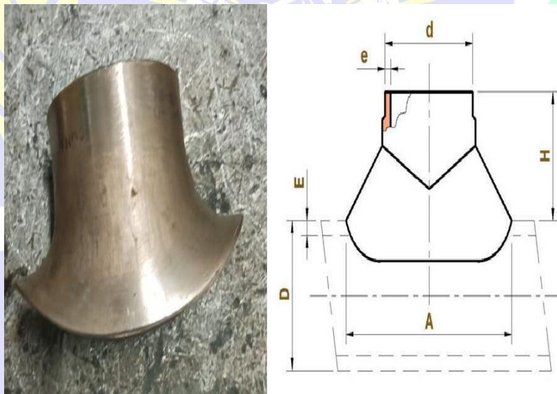
Gambar 8. Bentuk dan Model Material Saddle
