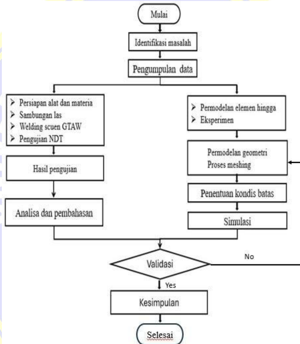
Gambar 5. Skema Diagram Alir
