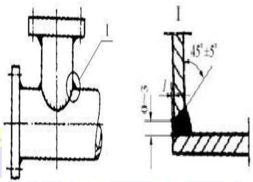
Gambar 9. Posisi Pengelasan
