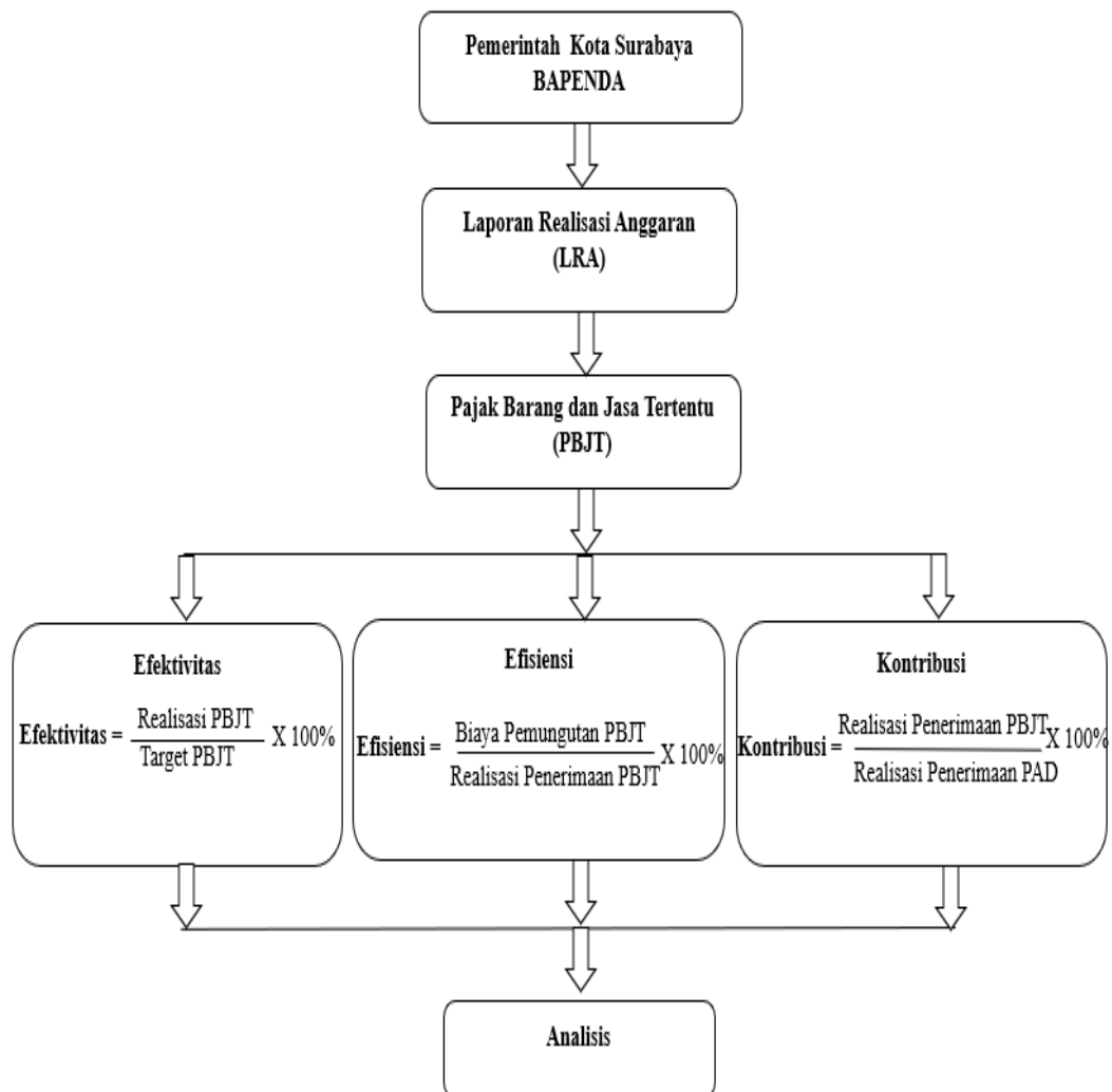
Gambar 2.1 Kerangka Berfikir
